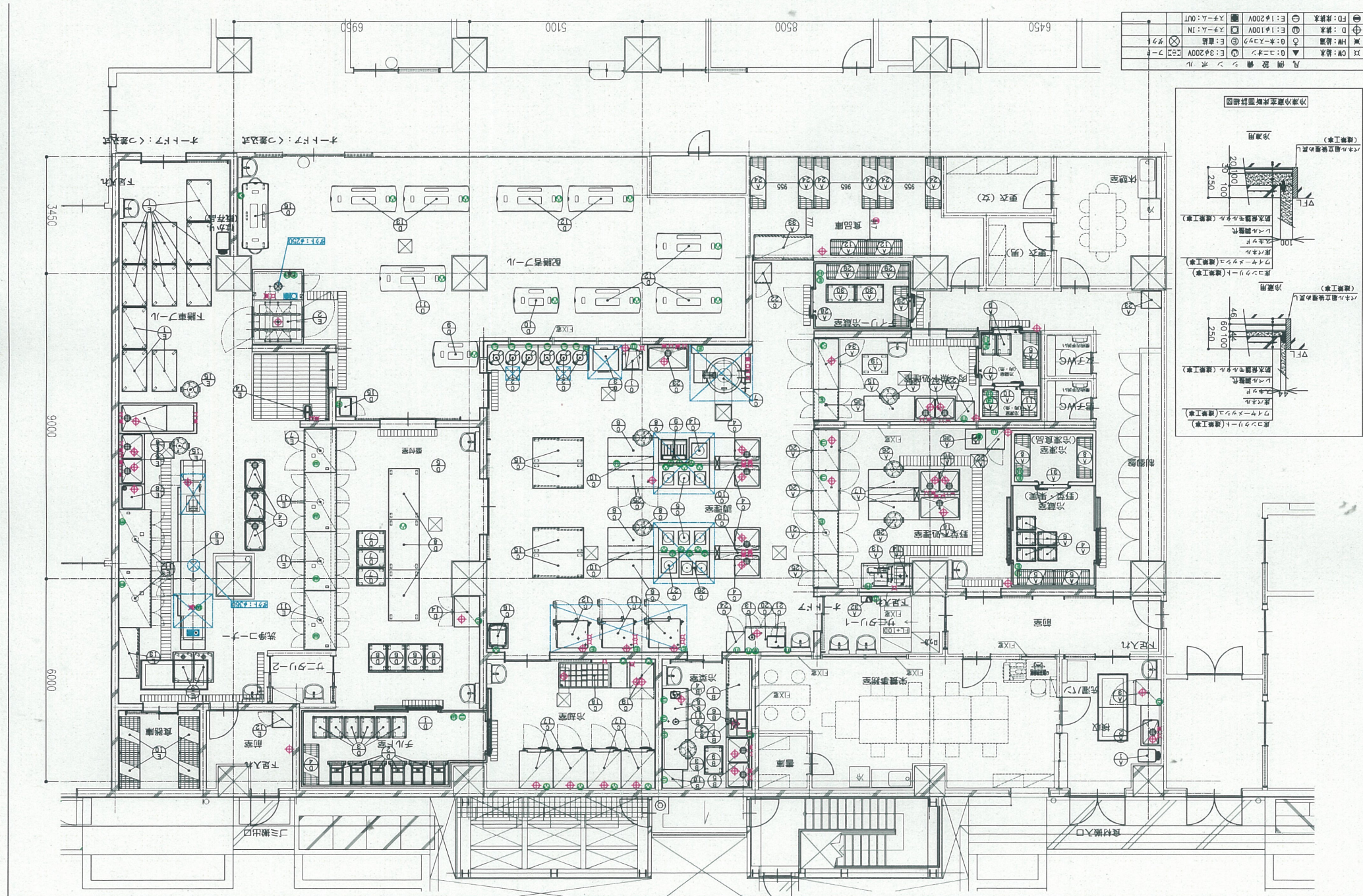
岡山市立市民病院調理室図面
